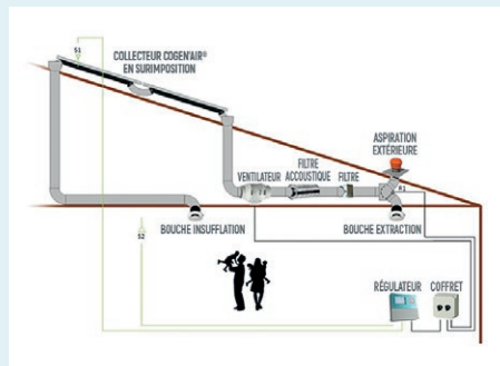
Fonctionnement de l'installation posée sous toit.
