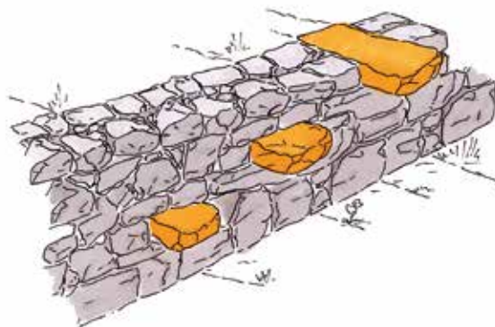
Deux exemples de franchissements couramment utilisés dans les pays de pierre sèche : moellons en saillie formant un escalier à claire voie et rampe (parfois pavée) « ouvrant » un mur.
